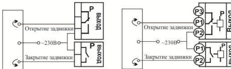
Подключение электрораздвижки
